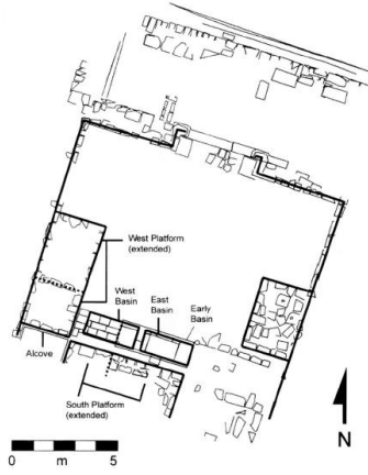
مخطط المعبد الصغير 1034
