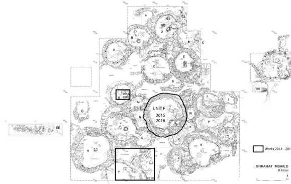
مخطط قرية اشكارا مسيعد 716
