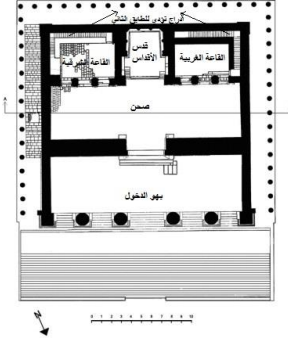
صورة لمعبد قصر البنت ومخططه (تصوير الباحث)
