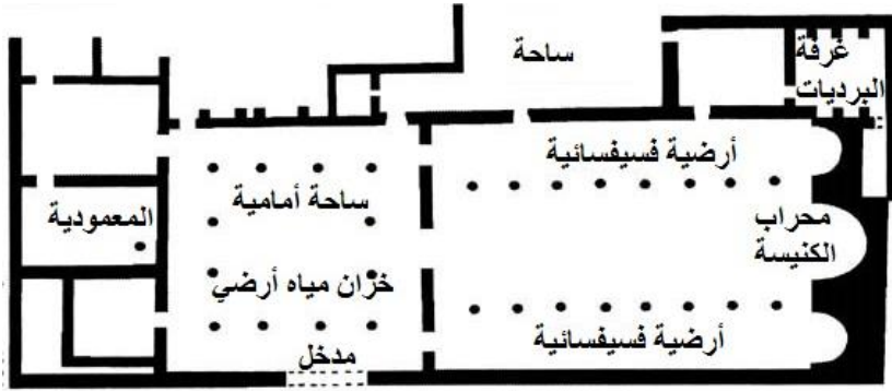
مخطط الكنيسة (إعداد الباحث)
