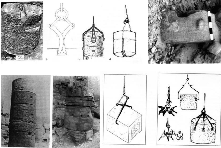
طريقة رفع أسطوانات الأعمدة 618
