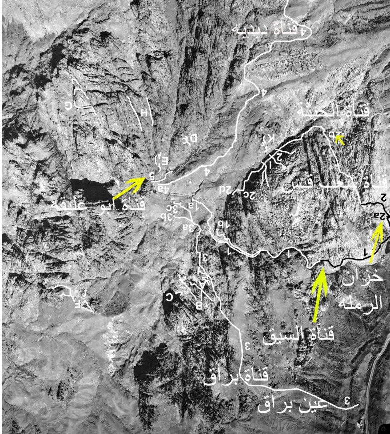
توزيع قنوات المياه النبطية داخل مدينة البتراء 837
