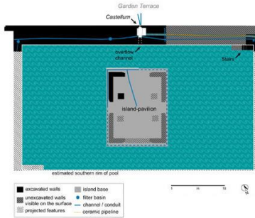
موقع الحديقة ومخططها 1037
