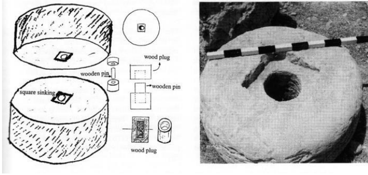
طريقة تثبيت أسطوانات الأعمدة فوق بعضها البعض 619
