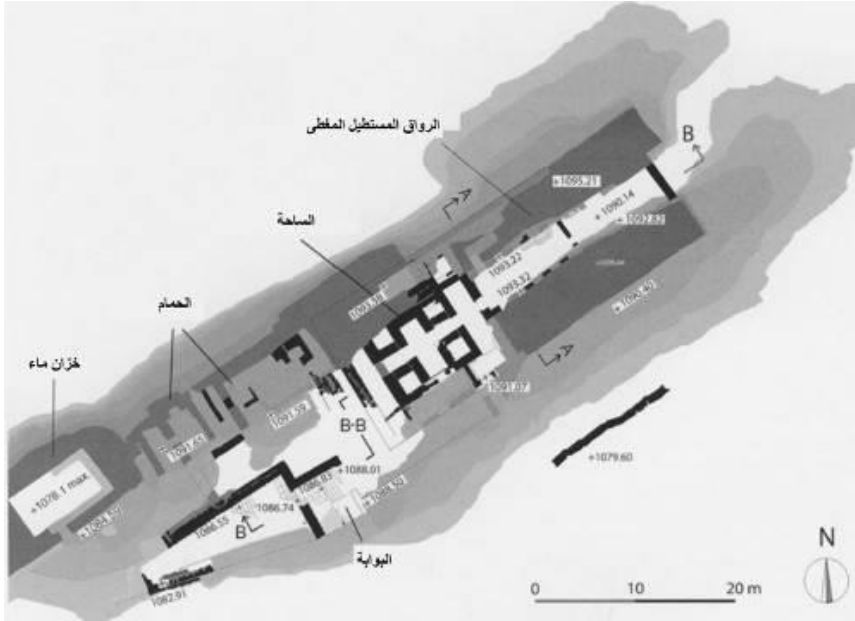
مخطط المنشأة المعمارية التي كُشف عنها في منطقة أم قُصَّه 1081
