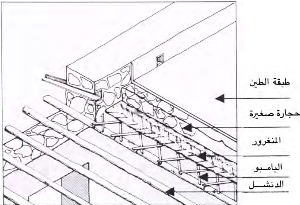
(لوحة رقم ٤٣) طريقة البناء بالمواد التقليدية
