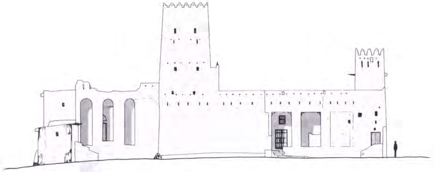
ELEVATION S-E
