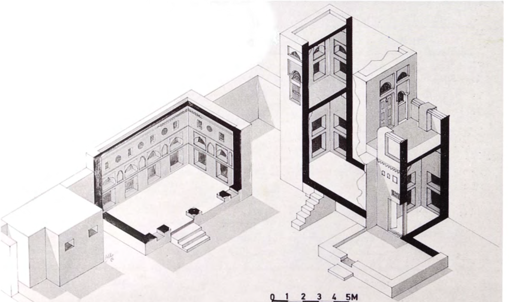
(لوحة رقم ٢٣) مجسم لبيت عبد الله بن سعد المطلق بالوكرة. المصدر: مركز التراث الشعبي لدول مجلس التعاون - الدوحة.
